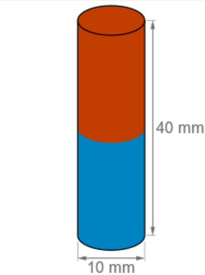
Måttritning · alla mått i mm
