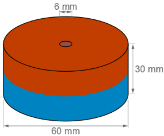
Måttitritning · alla mått i mm
