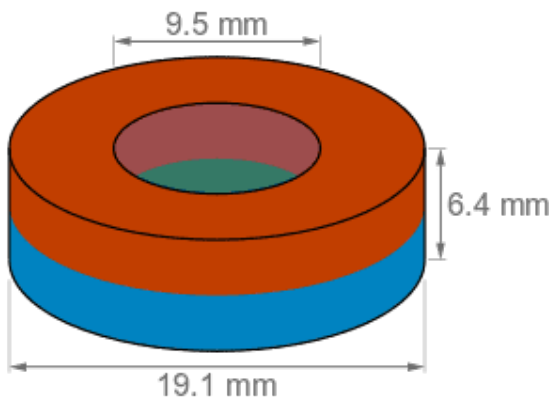
Mått ritning · alla mått i mm
