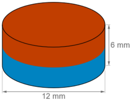
Måttritning · alla mått i mm
