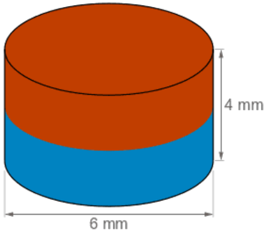
Måttitritning · alla mått i mm
